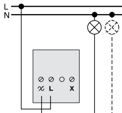
Поворотный светорегулятор с выключателем MTN5131-0000
