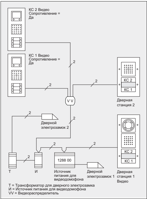
Пример аудио-/видеодомофонной системы. 2 дверные станции (лучевое соединение)
