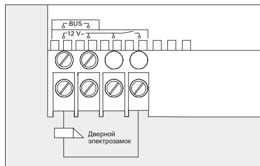
Подключение дверного электрозамка
