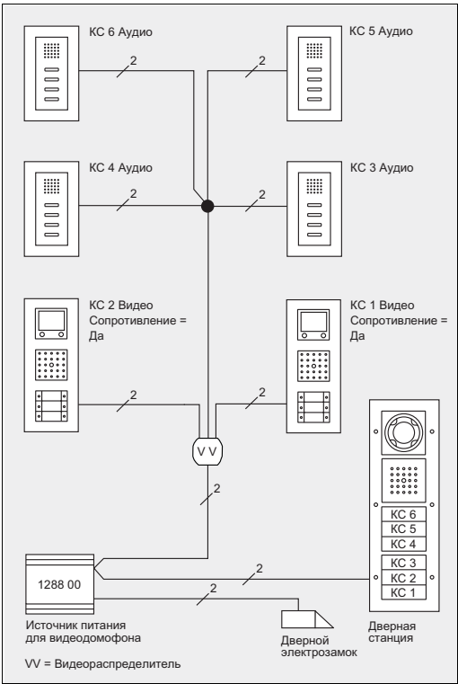
Пример аудио-/видеодомофонной станции. 6-квартирный дом (лучевое соединение с узлом развязки)
