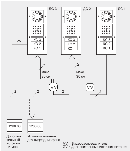
Пример видеодомофонной системы. Подключение нескольких дверных станций с цветными камерами
