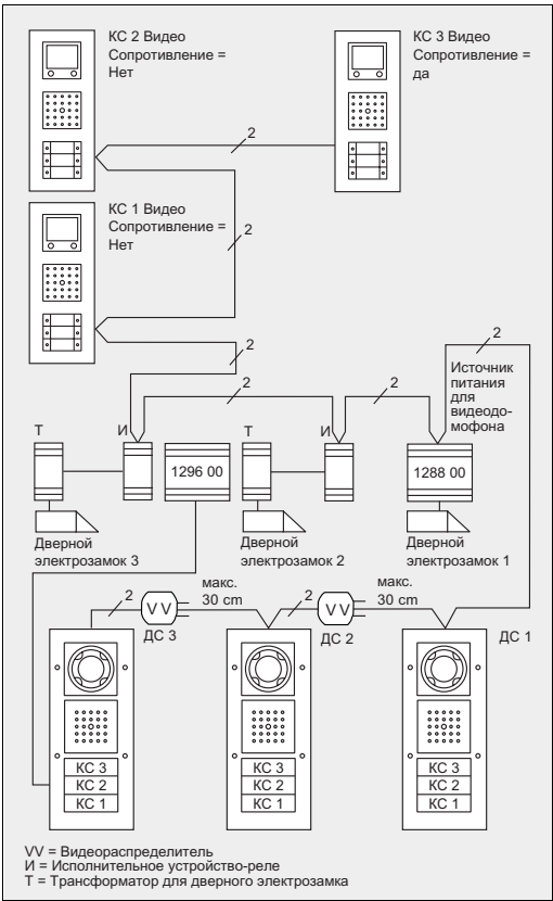
Пример видеодомофонной системы. Три дверные станции с цветными видеокамерами (шлейфовое соединение)
