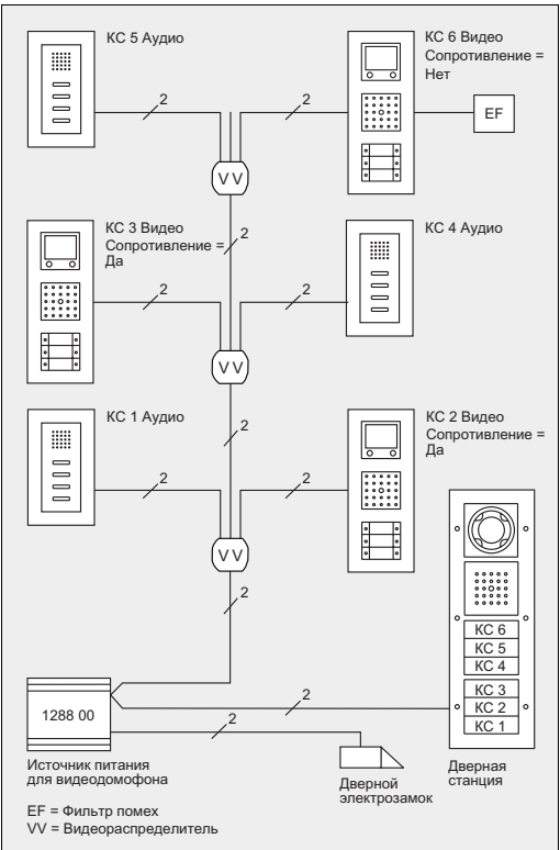
Пример аудио-/видеодомофонной системы. 6-квартирный дом (лучевое соединение)
