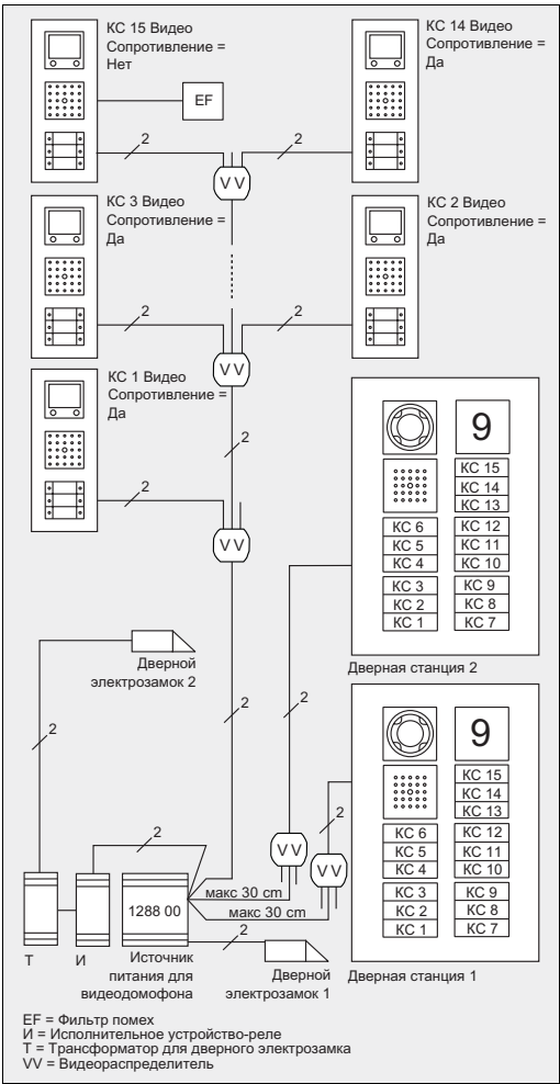
Пример видеодомофонной системы. Здание с пятнадцатью квартирными станциями (лучевое соединение)
