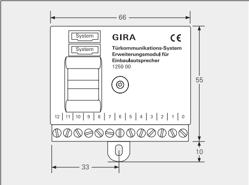
Габариты
