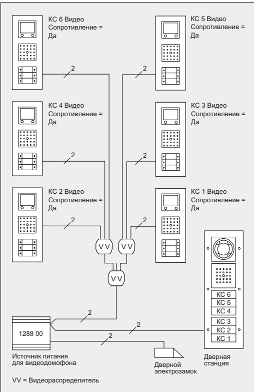
Пример видеодомофонной системы. 6-квартирный дом (звездообразная разводка)
