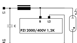
БЗУ для HI-ламп, напряжение зажигания 1,3 кВ
