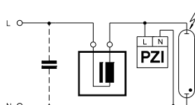
БЗУ для HI-ламп, напряжение зажигания 0,9 кВ
