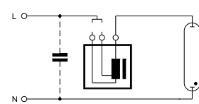
HS-лампы со встроенным устройством зажигания (ПРА с двумя альтернативными отводами напряжения)
