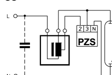
БЗУ для стандартных HS-ламп
