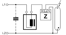
ИЗУ для HS- и HI-ламп в многофазные устройства питания
