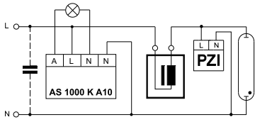
Пусковой переключатель для HI-ламп, напряжением зажигания 0,9 кВ
