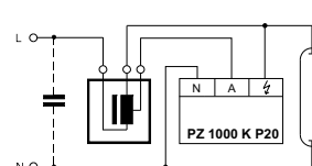
БЗУ для HS- и HI-ламп
