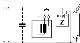
ИЗУ для HS- и HI-ламп (ПРА с двумя альтернативными отводами мощности)
