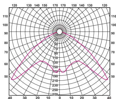
TL20WMH-02 КПД – 47%
