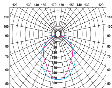
TL20WMH-01 КПД – 55%
