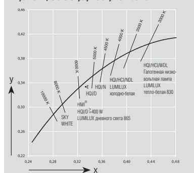
Фрагмент цветового графика с кривой Планка
