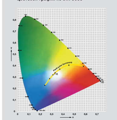
Цветовой график по DIN 5033
