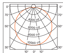
Полярная диаграмма
