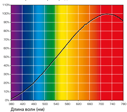
Рис. 5: Спектр галогенной зеркальной лампы: здесь равным образом представлены все цвета.
