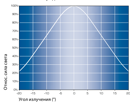
Рис. 4: Распределение света
