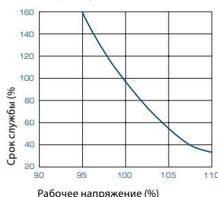
Влияние рабочего напряжения на срок службы
