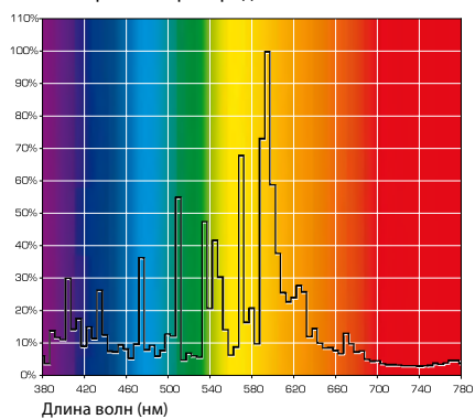
Рис. 6: Спектр газоразрядной лампы цвета „ww“ (белый теплый): смешение разных цветов образует белый цвет освещения с хорошей цветопередачей.
