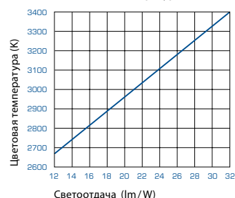
Взаимосвязь между светоотдачей и цветовой температурой
