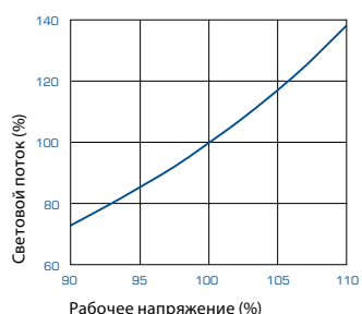
Влияние рабочего напряжения на световой поток
