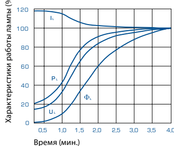
Рис. 1: Характеристические кривые пуска газоразрядной лампы
