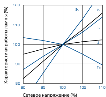
Рис. 2: Влияние изменения сетевого напряжения на характеристики работы газоразрядной лампы
