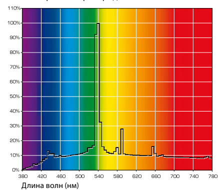
Рис. 7: Спектр лампы COLORLITE-зеленая: присутствует практически одна зеленая составляющая света.
