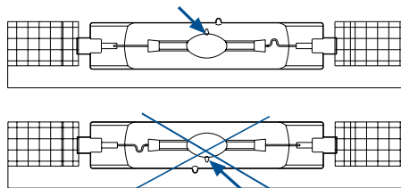
Рис. 4: Тепловой носик внутренней вакуумной колбы не должен быть направлен вниз.
