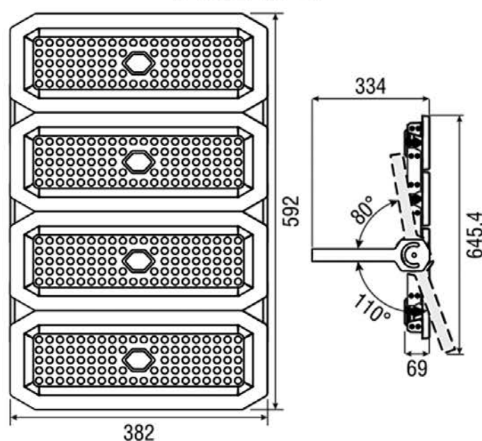
NFL-M2 400 Вт
