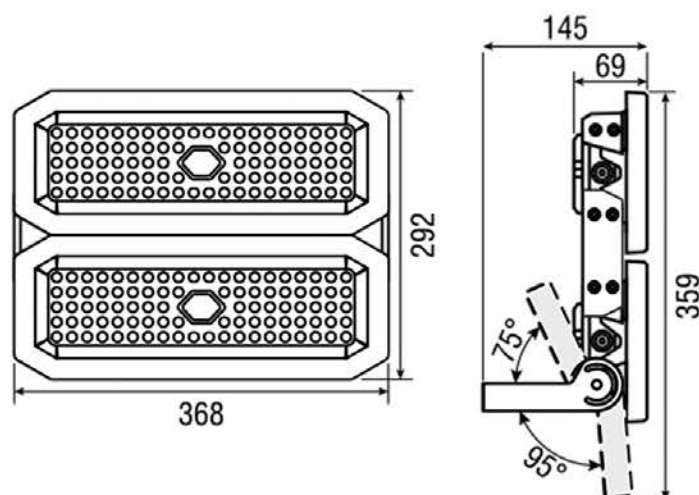
NFL-M2 150/200 Вт
