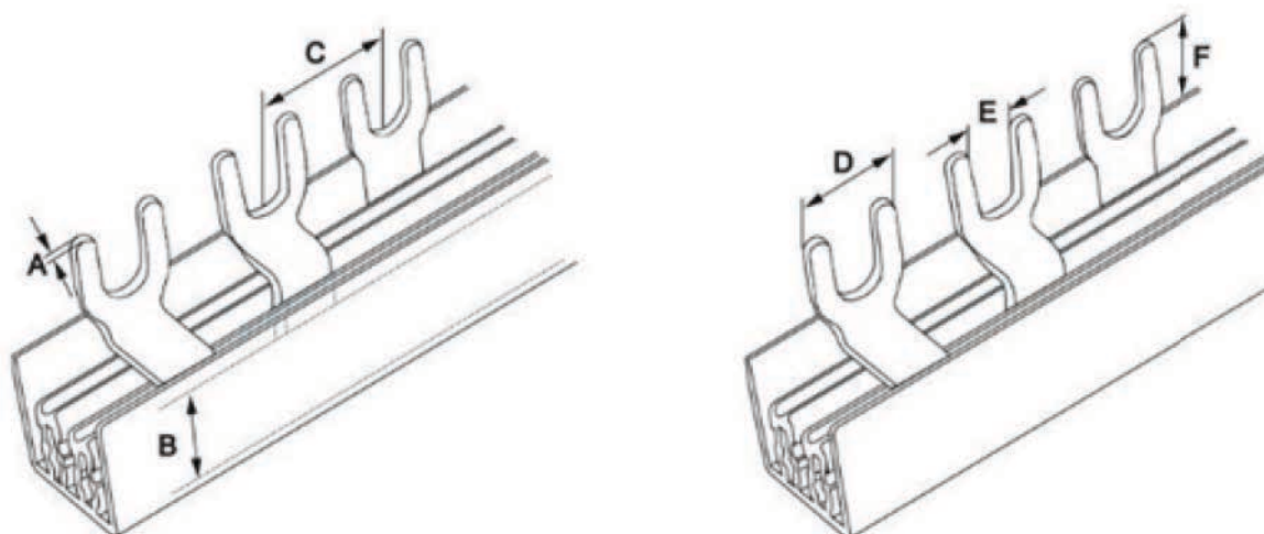
Рисунок 3 – Шина типа FORK 3P 63, 100 A
