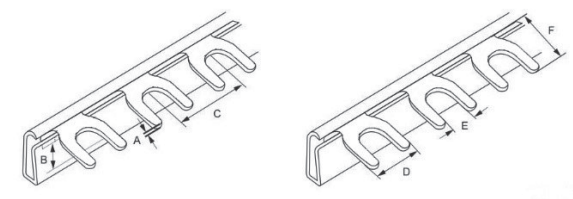
Шина типа FORK 1P 63, 100 А
