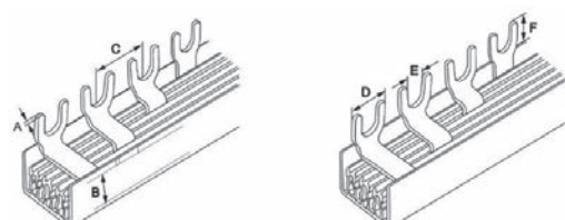
Шина типа FORK 4P 63, 100 А
