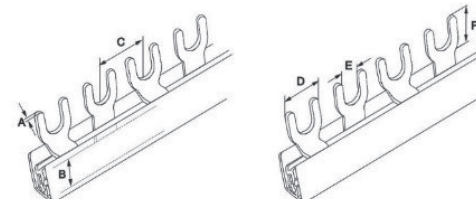
Шина типа FORK 2P 63, 100 А
