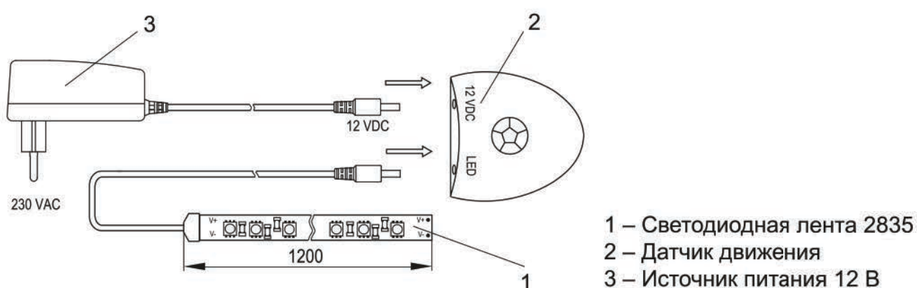
Рисунок 12 – Подключение комплекта LSR1-1-060-20-1-D12-S3
