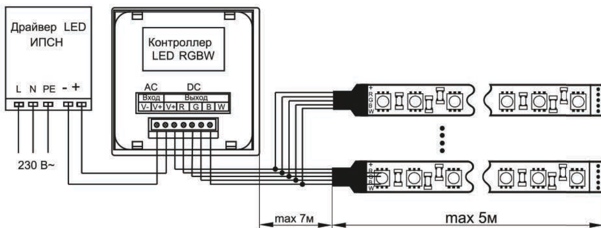
Рисунок 8 – Схема параллельного подключения многоцветной RGB, RGBW светодиодной ленты к блоку питания и контроллеру
