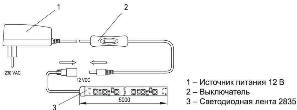
Рисунок 14 – Подключение LSR1-2-060-20-1-05-S1, LSR1-2-060-65-1-05-S1, LSR1-1-060-20-1-05-S1, LSR1-1-060-65-1-05-S1
