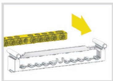
1.5.1 Крепление шины к суппорту Busbars mount to the support
