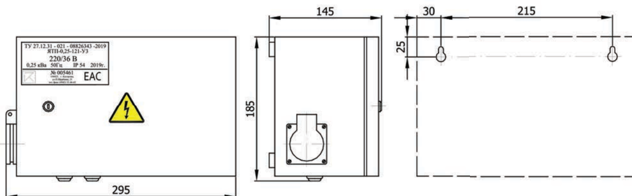
Рис.4 Габаритные размеры и масса
