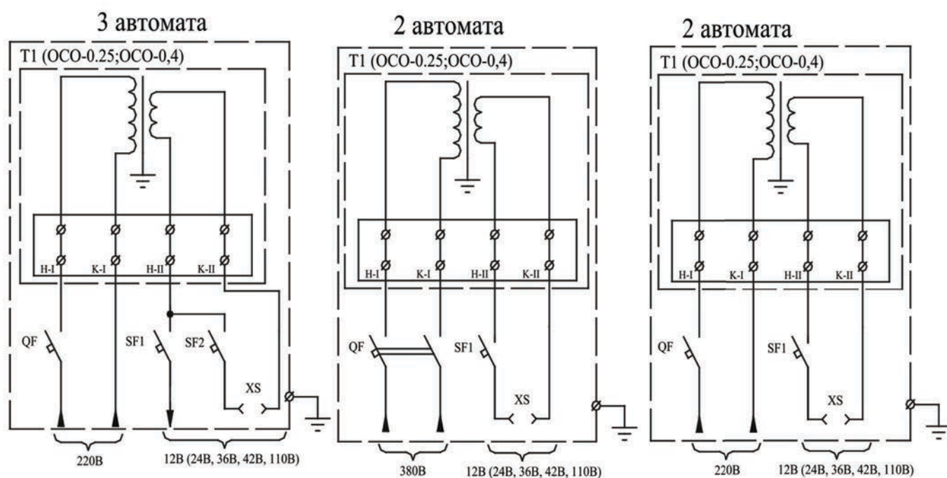
Рис.1 Схема электрическая принципиальная: ЯТП-0,25-220 УЗ IP-31; ЯТП -0,4-230 УЗ IP-31; ЯТП-0,25-230 УЗ IP-31; ЯТП -0,4-220 УЗ IP-31.
