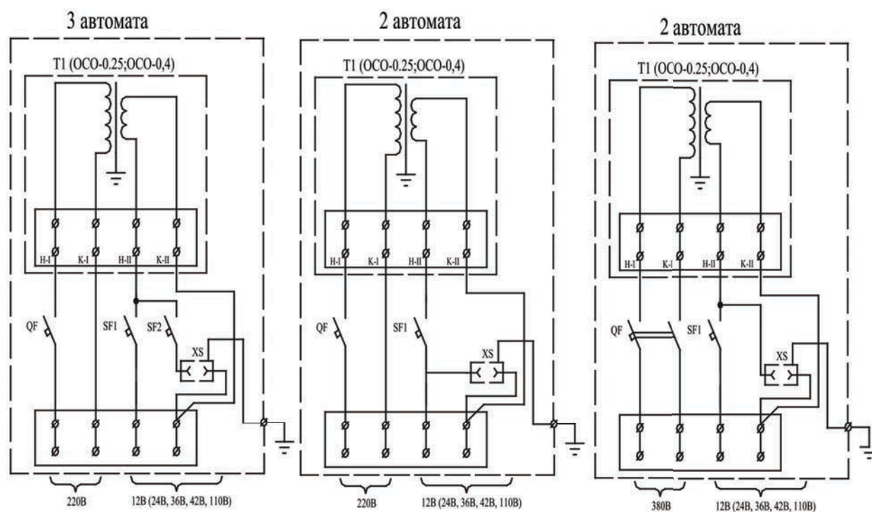
Рис.2 Схема электрическая принципиальная: ЯТП-0,25-121УЗ IP-54; ЯТП-0,4-131УЗ IP-54; ЯТП-0,25-131УЗ IP-54; ЯТП-0,4-121УЗ IP-54.
