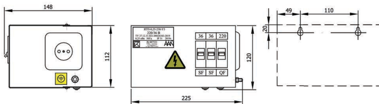
Рис.3 Габаритные размеры и масса
