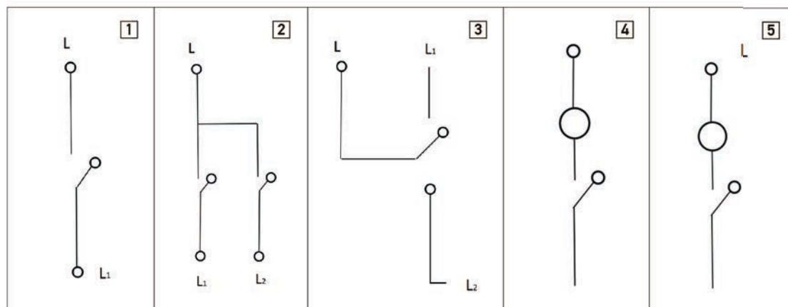
Рисунок 1. Электрические схемы выключателей серии DITA (TOKOV™):
