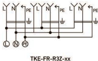
Рисунок 1. Электрические схемы розеток серии FREA (TOKOV™).
