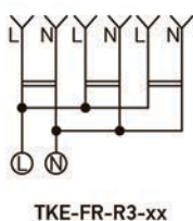
Рисунок 1. Электрические схемы розеток серии FREA (TOKOV™).
