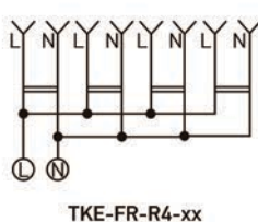
Рисунок 1. Электрические схемы розеток серии FREA (TOKOV™).
