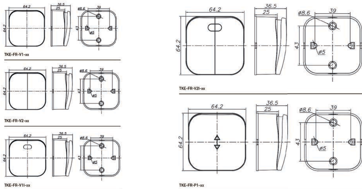
Рисунок 2. Габаритные размеры выключателей серии FREA (ТОКОВ™).
