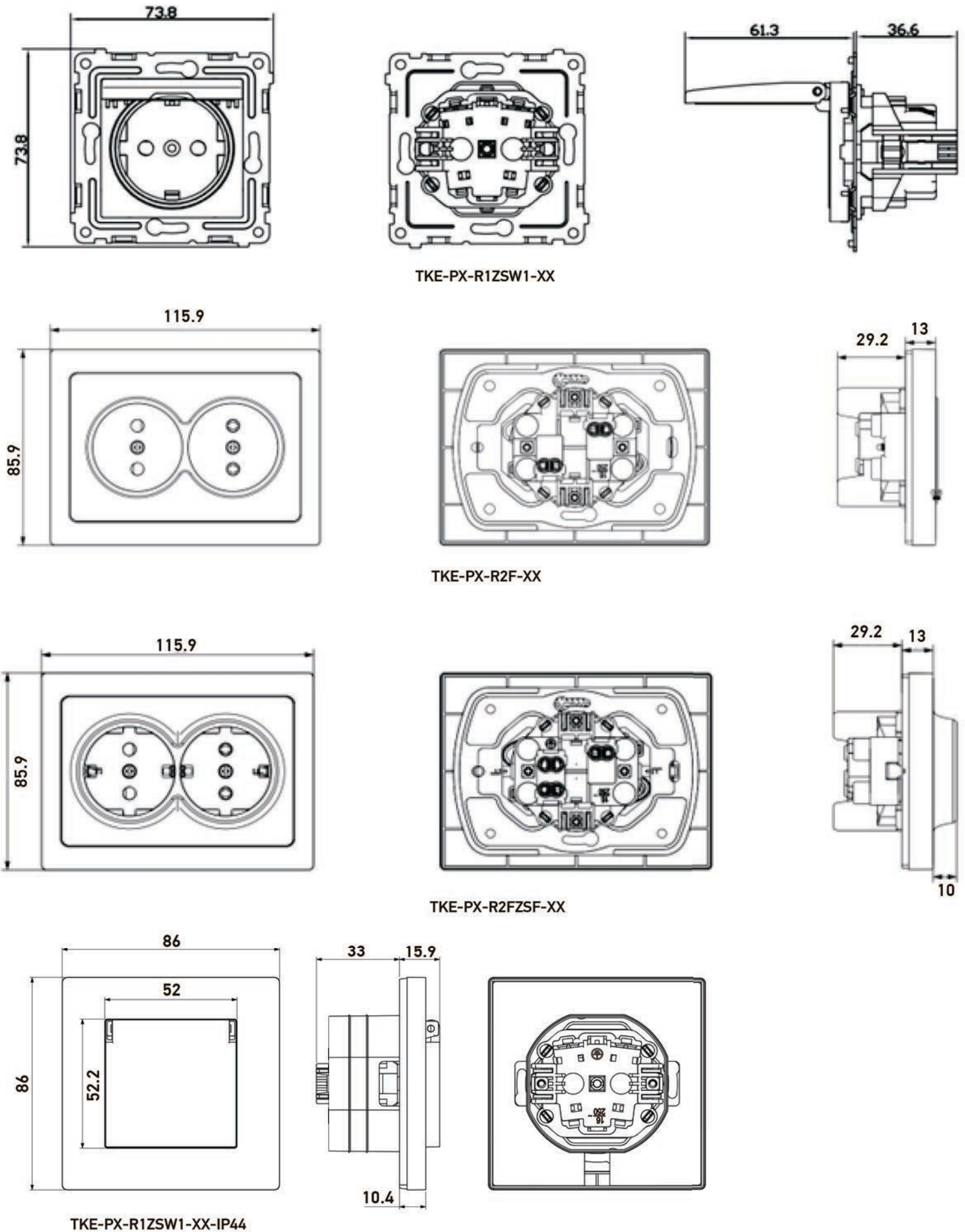
Рисунок 2. Габаритные размеры розеток серии PIXEL (ТОКОВ™).
