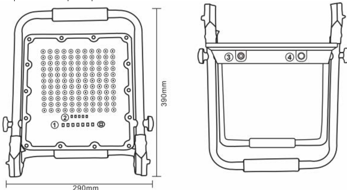
1 – Сигнальный (проблесковый) маячок оранжевого цвета; 2 – светодиодный индикатор уровня заряда аккумуляторной батареи; 3 – разъем для подключения зарядного устройства 5В/2А; 4 – кнопка включения/переключения режимов/выключения.
