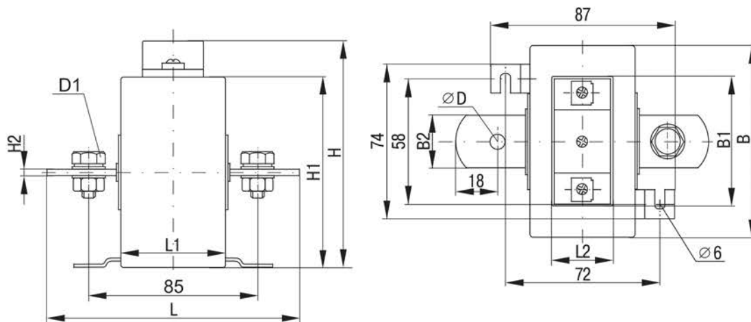
Рисунок 1 – Габаритные и установочные размеры трансформаторов ТОП-0,66
