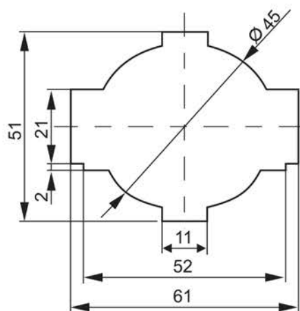
ТШП-0,66 габарит 60
