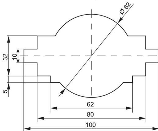
ТШП-0,66 габарит 100
