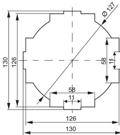
ТШП-0,66 габарит 125
