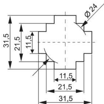
ТШП-0,66 габарит 30
