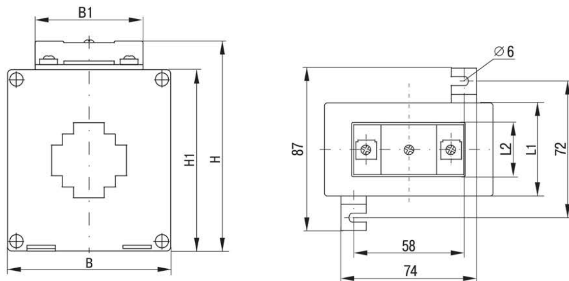
б) модификации ТШП-0,66 габарит 30(Т)
