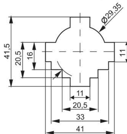
ТШП-0,66 габарит 40
