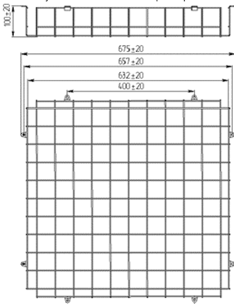
Рисунок 2. Чертеж решётки
