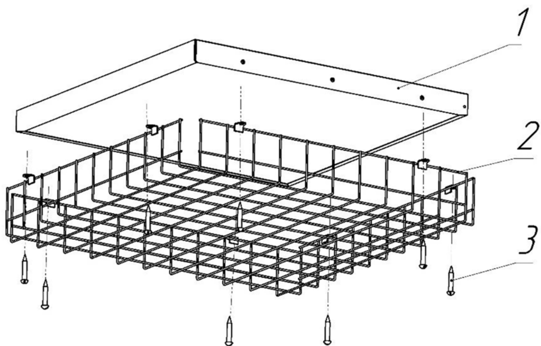
Рисунок 1. Схема монтажа защитной решётки
