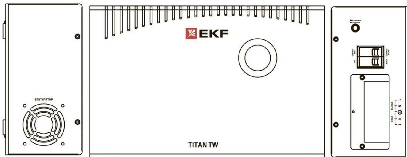
Рис. 2 Внешний вид стабилизатора TW-3000-10000
