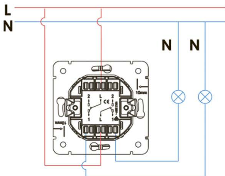
1-, 2-клавишный проходной 1, 2 gang 2 way switch
