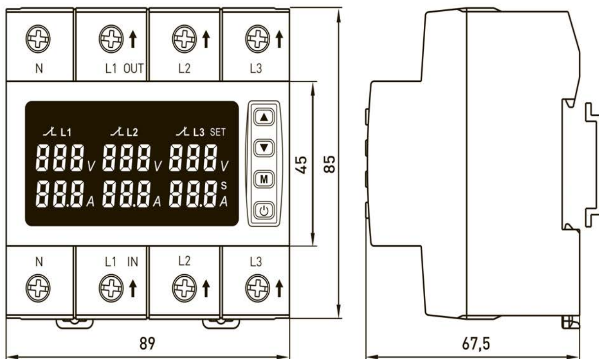
Рисунок 4. Габаритные и установочные размеры изделия
