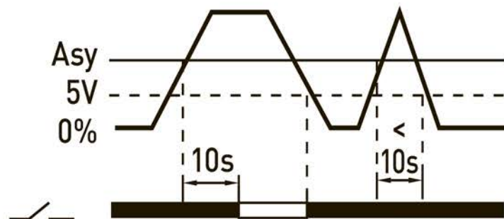
Рисунок 3. Диаграмма работы реле при превышении установленного значения порога срабатывания при асимметрии
