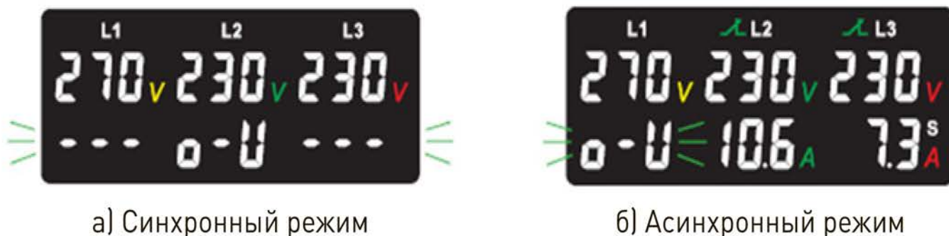
Рисунок 10. Внешний вид дисплея в случае повышенного напряжения на фазе L1
