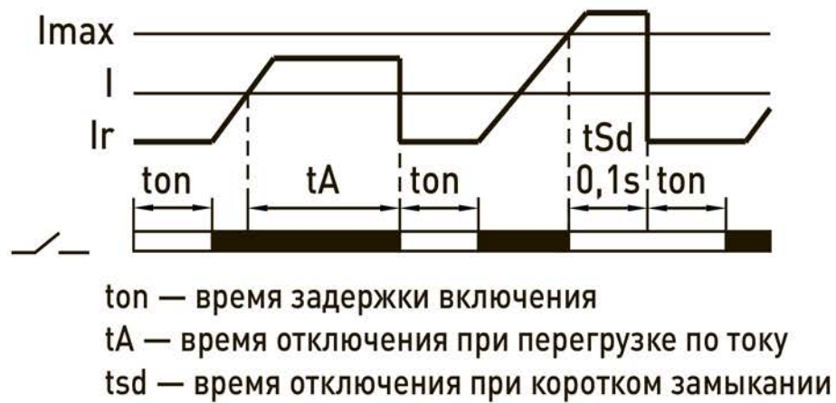
Рисунок 2. Диаграмма работы реле при превышении установленного значения тока
