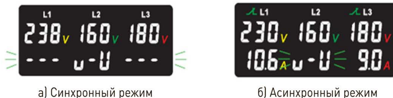
Рисунок 11. Внешний вид дисплея в случае пониженного напряжения на фазе L1
