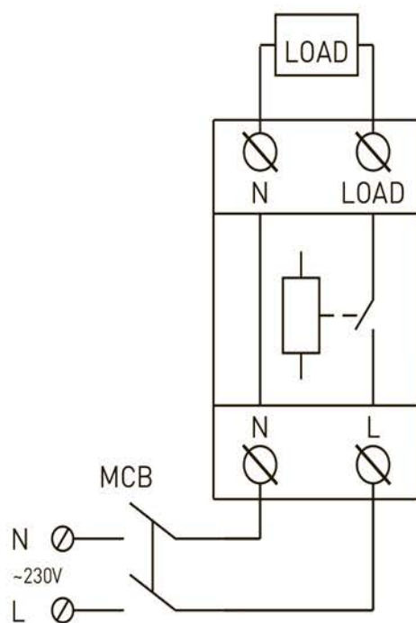
Рисунок 5. Схема электрическая подключения реле
