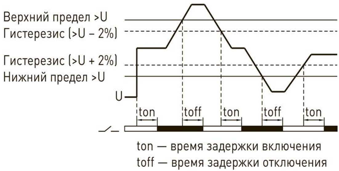
Рисунок 1. Диаграмма работы реле при выходе напряжения за установленные пределы
