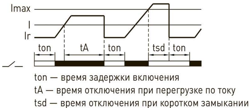
Рисунок 2. Диаграмма работы реле при превышении установленного значения тока
