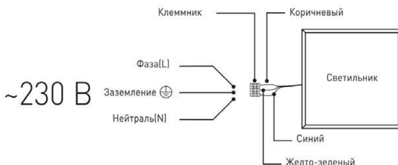
Рис.1. Схема подключения светильника к сети 230В.
