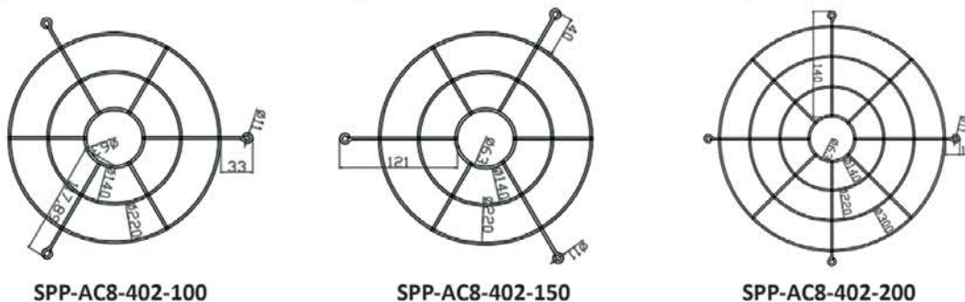
Рис.1 Габаритные размеры решеток для светильников SPP-402 100 Вт, 150 Вт, 200 Вт.
