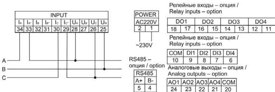
б) схема подключения мультиметра LCD к трехпроводной сети при I \leq 5 A, U \leq 600 В / LCD multimeter connection diagram to a three-wire network at I \leq 5 A, U \leq 600 V
