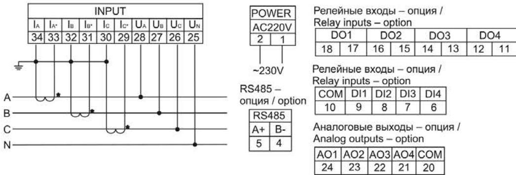
с) схема подключения мультиметра LCD к четырехпроводной сети при I > 5 A, U \leq 600 В / wiring diagram of the multimeter LED, LCD to a four-wire network at I > 5 A, U \leq 600 V
