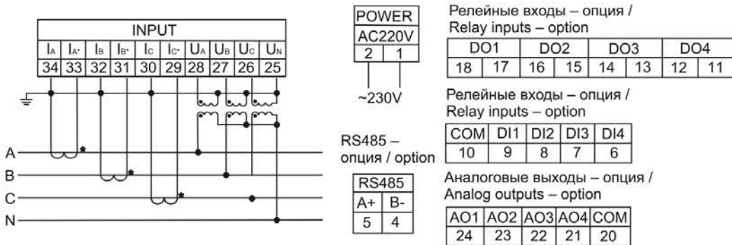
е) схема подключения мультиметра LCD к четырехпроводной сети при I > 5 A, U > 600 В / LCD multimeter connection diagram to a four-wire network at I > 5 A, U > 600 V
