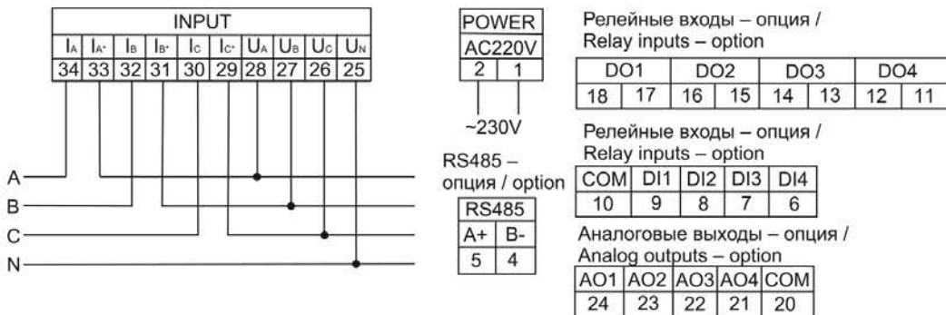
а) схема подключения мультиметра LCD к четырехпроводной сети при I \leq 5 A, U \leq 600 В / LCD multimeter connection diagram to a four-wire network at I \leq 5 A, U \leq 600 V
