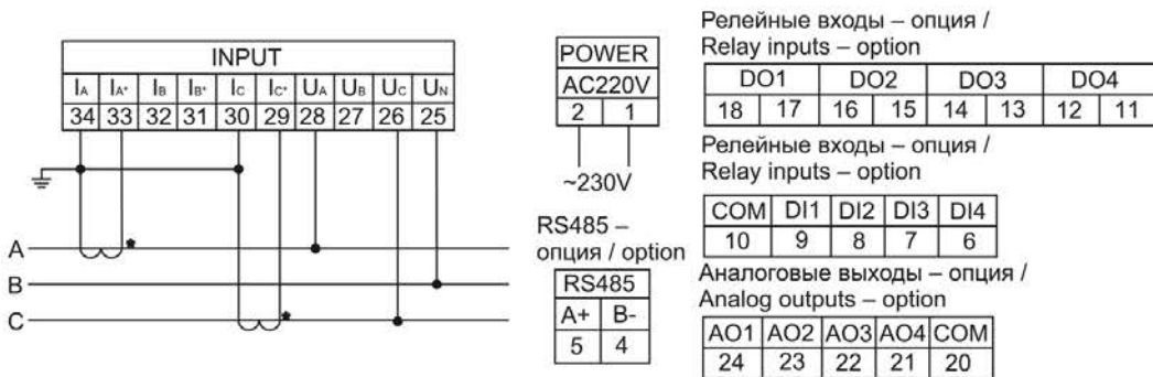
д) схема подключения мультиметра LCD к трехпроводной сети при I > 5 A, U \leq 600 В / wiring diagram of the multimeter LED, LCD to a three-wire network at I > 5 A, U \leq 600 V
