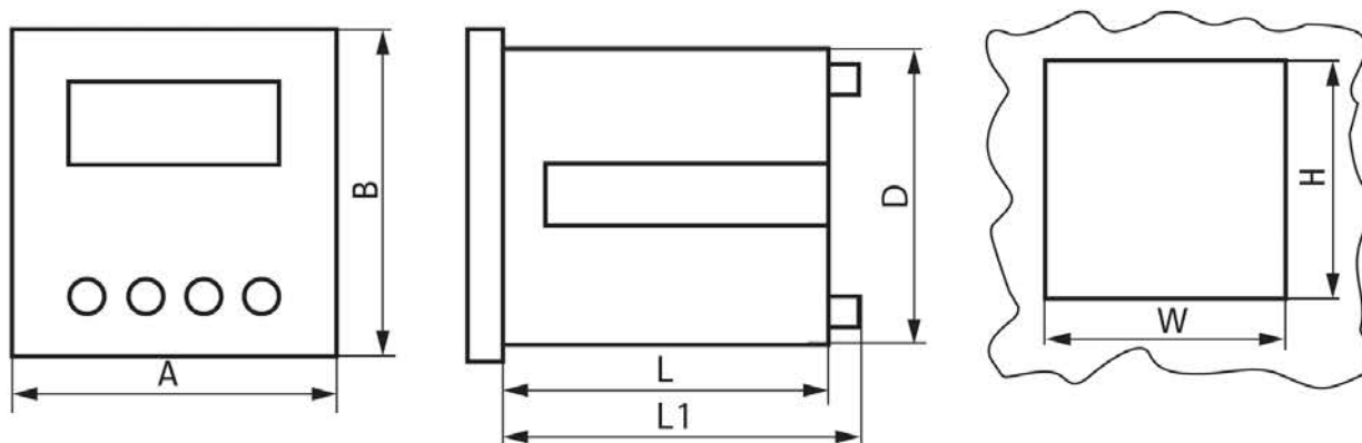
Рис. 2 Габаритные размеры
