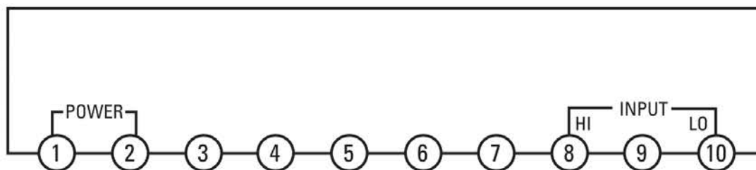
Рис. 8 Обозначение клемм для приборов размером 96x96
