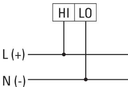
Рис.3 Схема подключения вольтметра при U \leq 500\text{В}
