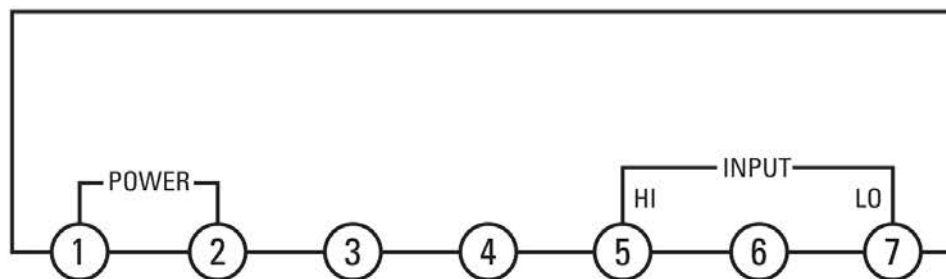
Рис. 7 Обозначение клемм для приборов размером 72x72
