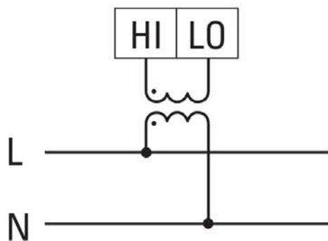
Рис.4 Схема подключения вольтметра при U > 500V
