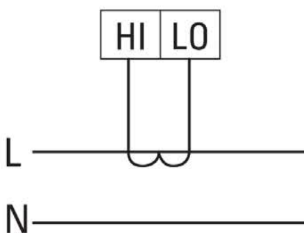
Рис.6 Схема подключения амперметра при I > 5A
