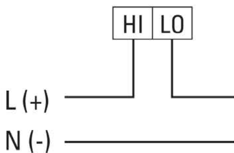
Рис.5 Схема подключения амперметра при I \leq 5A
