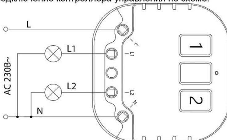
Рис. 1 Схема подключения LD313
