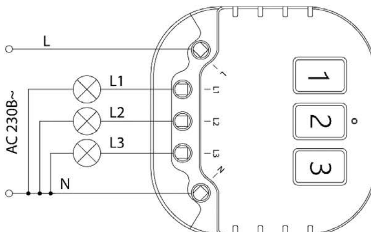
Рис. 2 Схема подключения LD314
