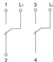
д) выключатель двухклавишный проходной / pass-through 2-gang switch / екі пернелі өтпелі ажыратқыш / intrerupator dublu de trecere prin / indikatsiyali ikkita klavishli viklyuchatel
