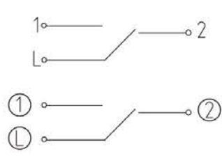
11) выключатель двухклавишный проходной / pass-through 2-gang switch / екі пернелі өтпелі ажыратқыш
