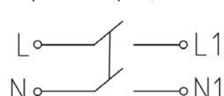
8) выключатель одноклавишный двухполюсный / 2-pole 1-gang switch / екі полюсті бір пернелі ажыратқыш
