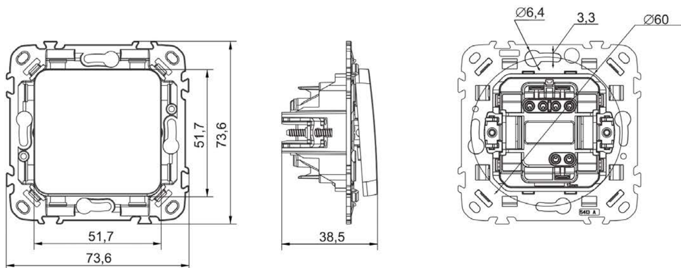
Рисунок 2 – Габаритные и установочные размеры одноклавишных выключателей /
