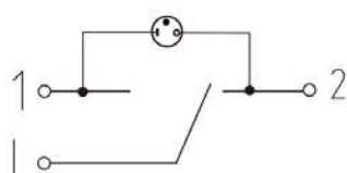
7) выключатель одноклавишный проходной с индикацией / pass-through 1-gang switch with indication / индикациясы бар бір пернелі өтпелі ажыратқыш
