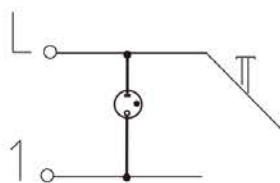
15) выключатель одноклавишный кнопочный с индикацией / 1-gang push-button switch with indication / индикациясы бар бір пернелі түймелі ажыратқыш
