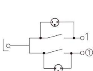
13) выключатель двухклавишный с индикацией / 2-gang switch with indication / индикациясы бар екі пернелі ажыратқыш
