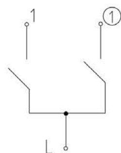
12) выключатель жалюзи с блокировкой / blind switch with lock / блокировкасы бар пердешелер ажыратқыш
