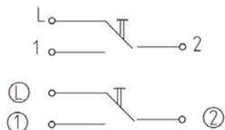
18) выключатель двухклавишный кнопочный проходной / pass-through 2-gang push-button switch / екі пернелі өтпелі түймелі ажыратқыш
