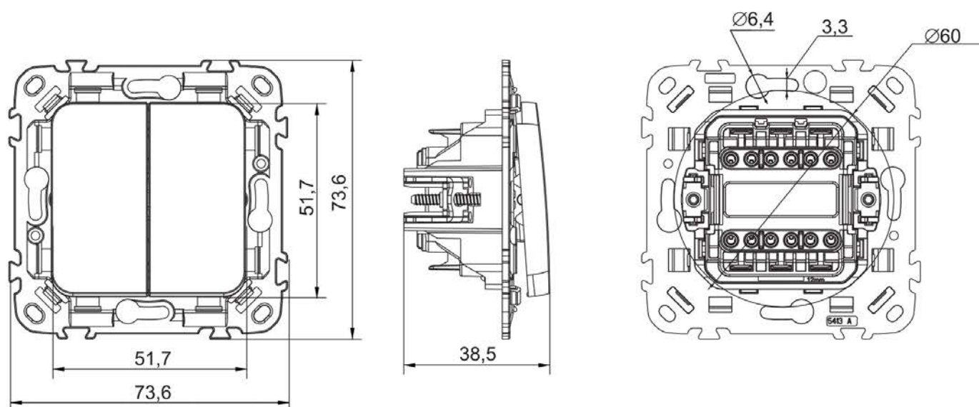
Рисунок 3 – Габаритные и установочные размеры двухклавишных выключателей /
