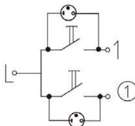
19) выключатель двухклавишный кнопочный с индикацией / 2-gang push-button switch with indication / индикациясы бар екі пернелі түймелі ажыратқыш
