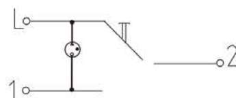
16) выключатель одноклавишный кнопочный проходной с индикацией / pass-through 1-gang push-button switch with indication / индикациясы бар бір пернелі өтпелі түймелі ажыратқыш
