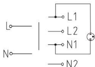
9) выключатель одноклавишный проходной двухполюсный с индикацией / pass- through 2-pole 1-gang switch with indication / индикациясы бар екі полюсті бір пернелі өтпелі ажыратқыш
