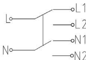
23) выключатель одноклавишный проходной двухполюсный / pass-through 2-pole 1-gang switch / екі полюсті бір пернелі өтпелі ажыратқыш
