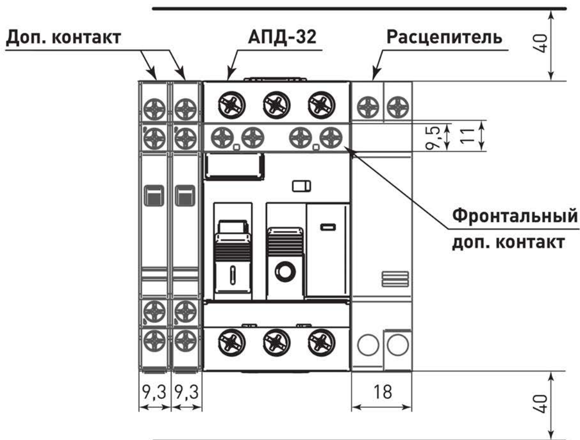
Рис. 9 – Габаритные размеры АД-32
