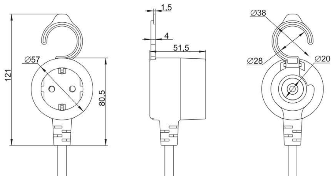
УШ-01М / USH-01M
