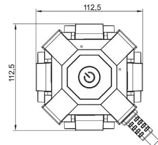
УШ-01М / USH-01M
