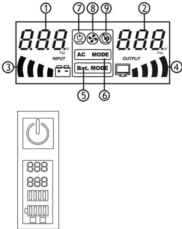
Рисунок 2 – Дисплей ИБП серии ELACTRA ET
