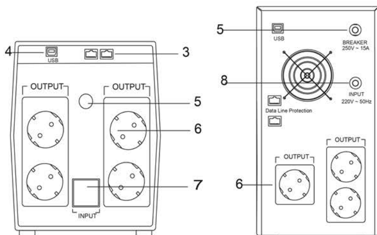
Рисунок 4 – Задняя панель ИБП серии ELACTRA ET
