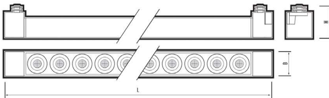
Рис.1 Прожектор PTR 42
