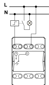
Кнопочный выключатель
