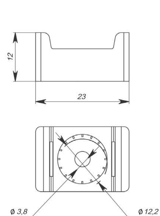
Рисунок 1 — Габаритные размеры Издание 1
