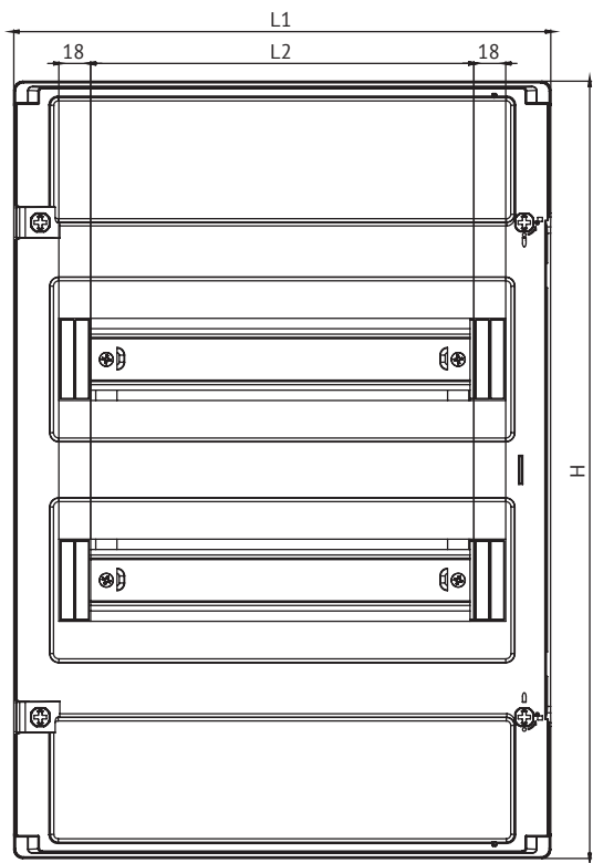
Вид спереди
