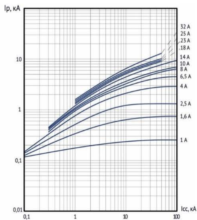
Рисунок В.4 – Характеристика зависимости тока отсечки от ожидаемого тока MP-32RH, MP-32RHI
