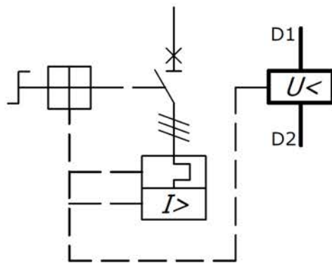
Рисунок Б.8 – Расцепитель минимального напряжения МР-У
