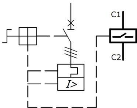
Рисунок Б.7 – Расцепитель независимый МР-А
