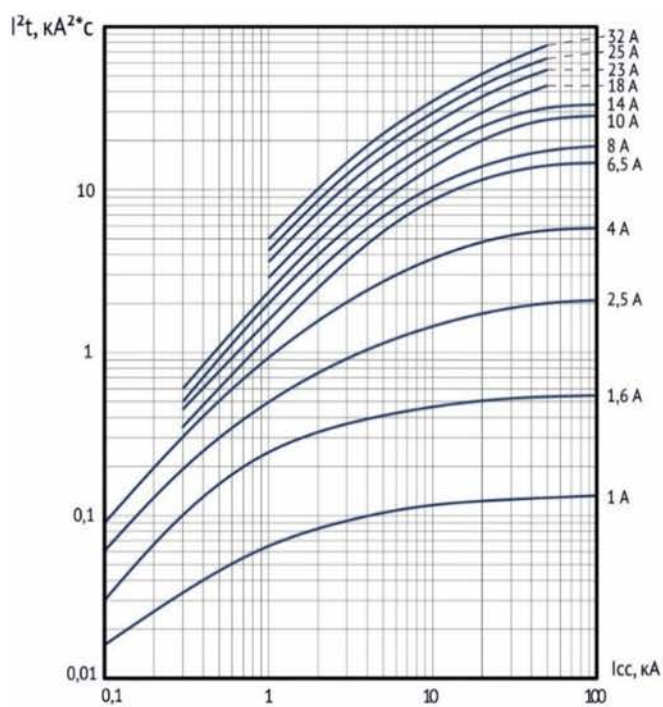
Рисунок В.3 – Характеристика I^2t MP-32RH, MP-32RHI
