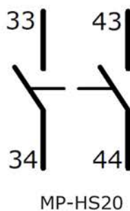
Рисунок Б.4 – Блоки контактные вспомогательные MP-HS
