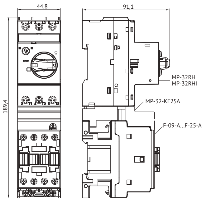
Сборка MP-32RH(I)...-T2 + MP-32-KF25A-T2 + F-09-A...F-25-A
