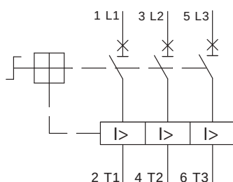
Автоматические выключатели MP-32RHI...-T2
