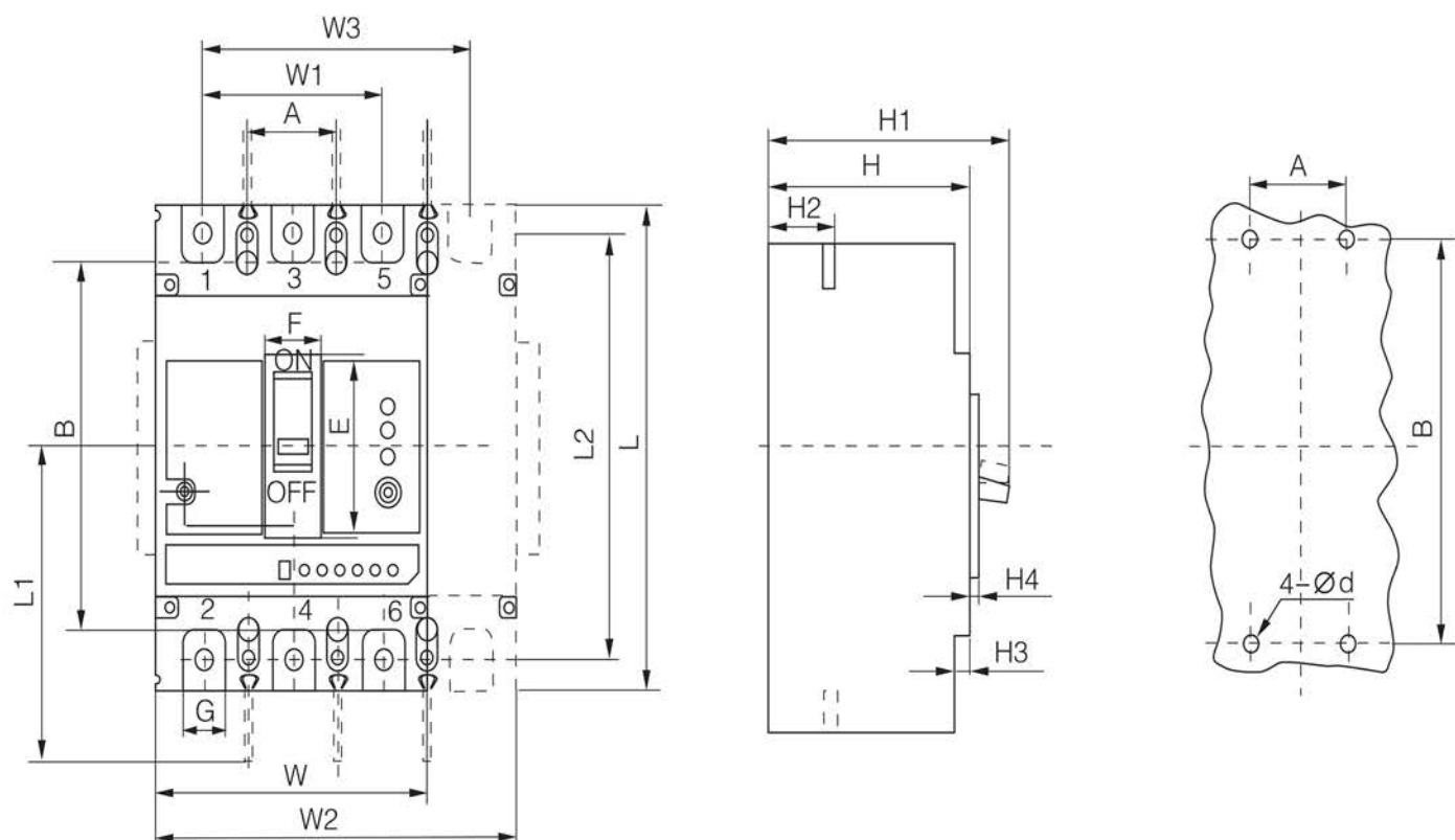
Габаритные размеры BA-99M 100, BA-99M 250, BA-99M 400, BA-99M 630-800 с электронным распределителем
