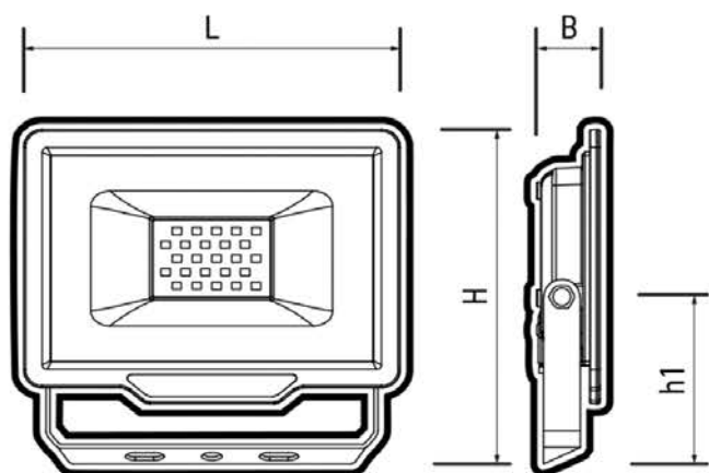
Рис. 1 Проектор PFL-C3
