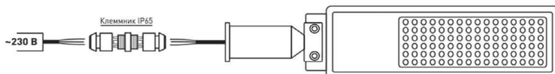
Рис.1. Схема подключения светильника к сети 230В.
