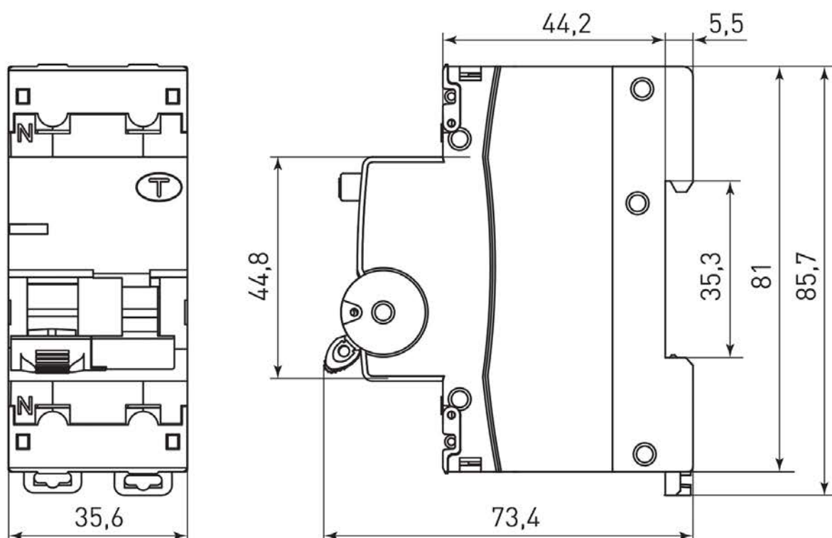
Рис. 3а – Габаритные размеры АВДТ-63N 1Р+N
