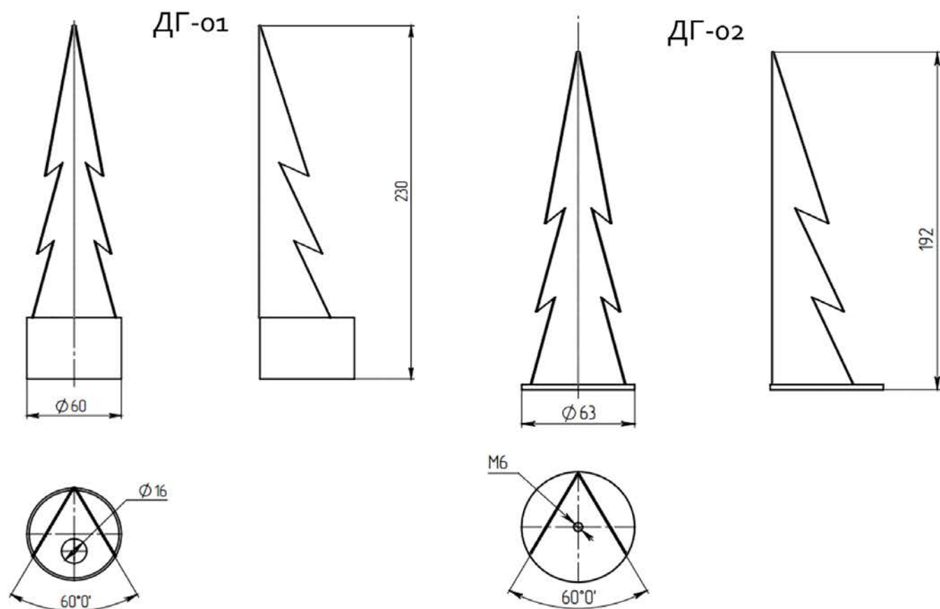
Рисунок 1. Общий вид держателей ДГ-01 и ДГ-02
