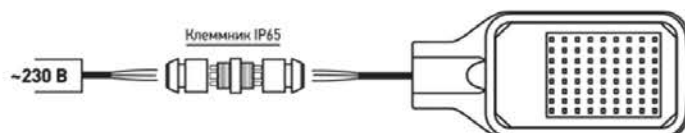
Рис.1. Схема подключения светильника к сети 230В.
