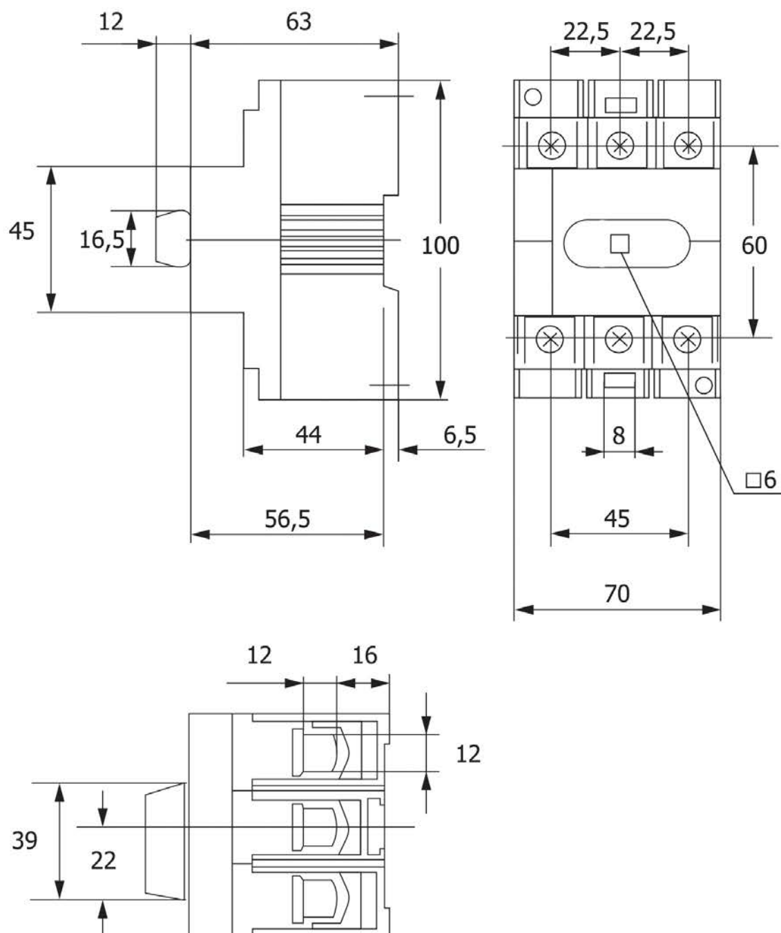
Рис. 1 – Габаритные и установочные размеры рубильников 40-125 А 3Р
