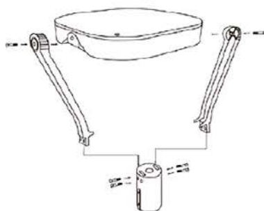
Рис.1. Схема сборки светильника.
