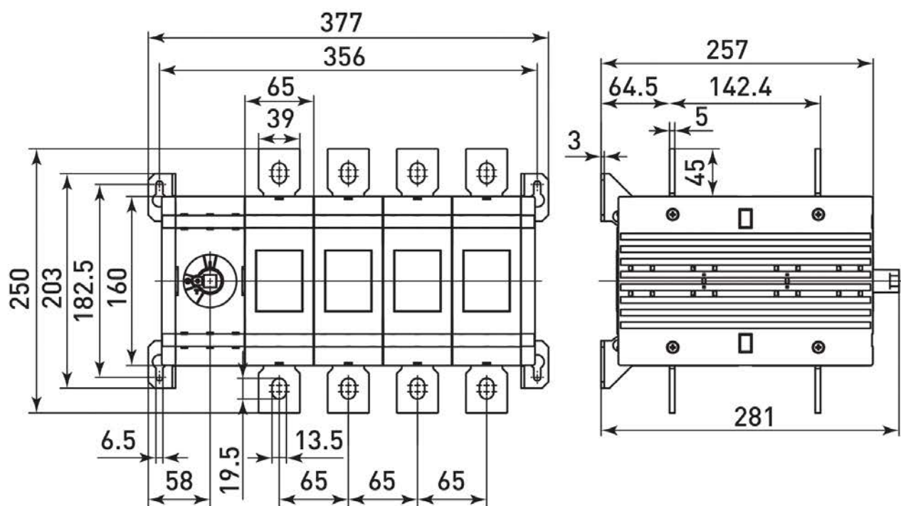
Рис. 18 – Габаритные и установочные размеры реверсивных рубильников 630-800 А 4Р
