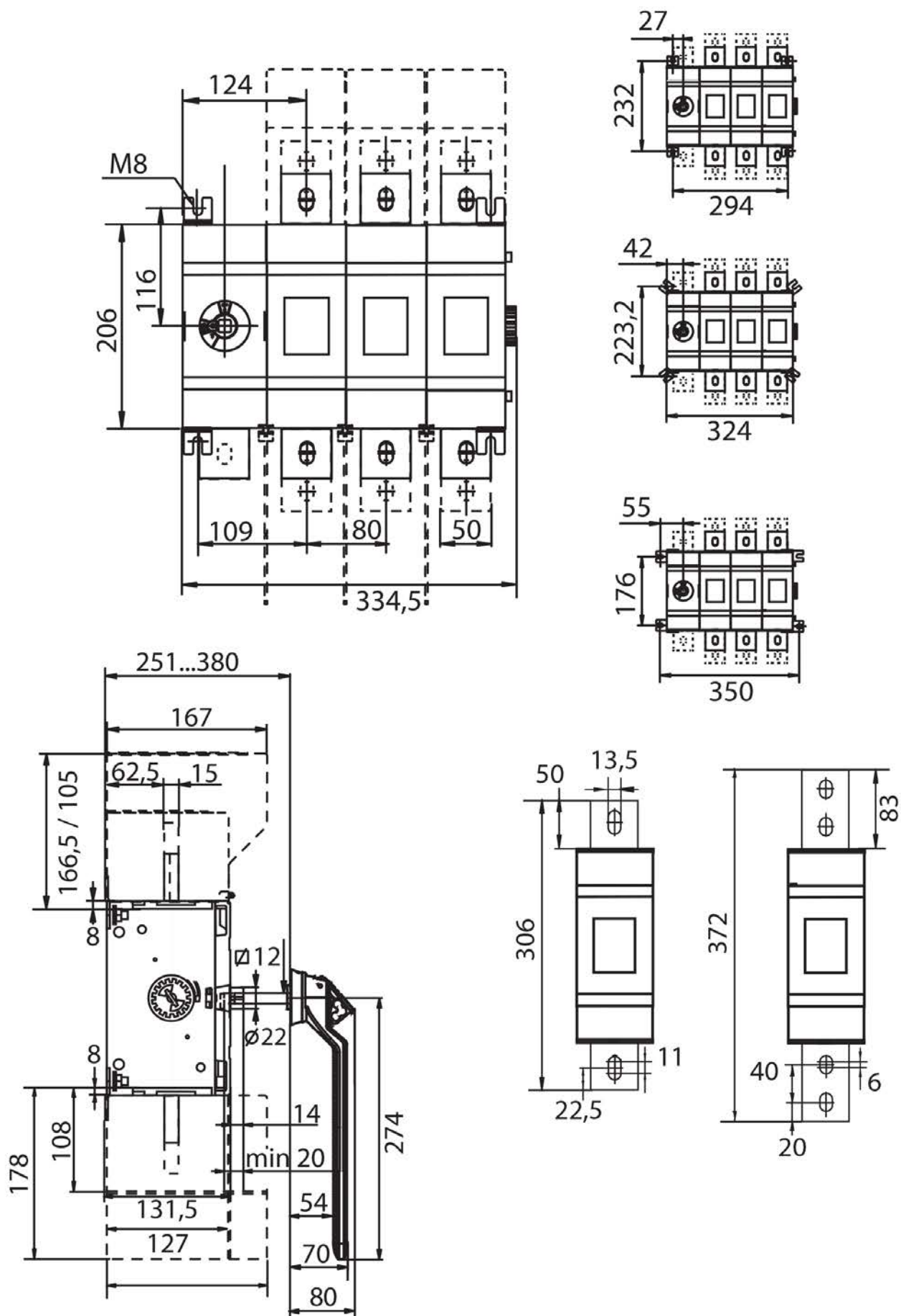
Рис. 8 – Габаритные и установочные размеры рубильников 1000-1600 А ЗР
