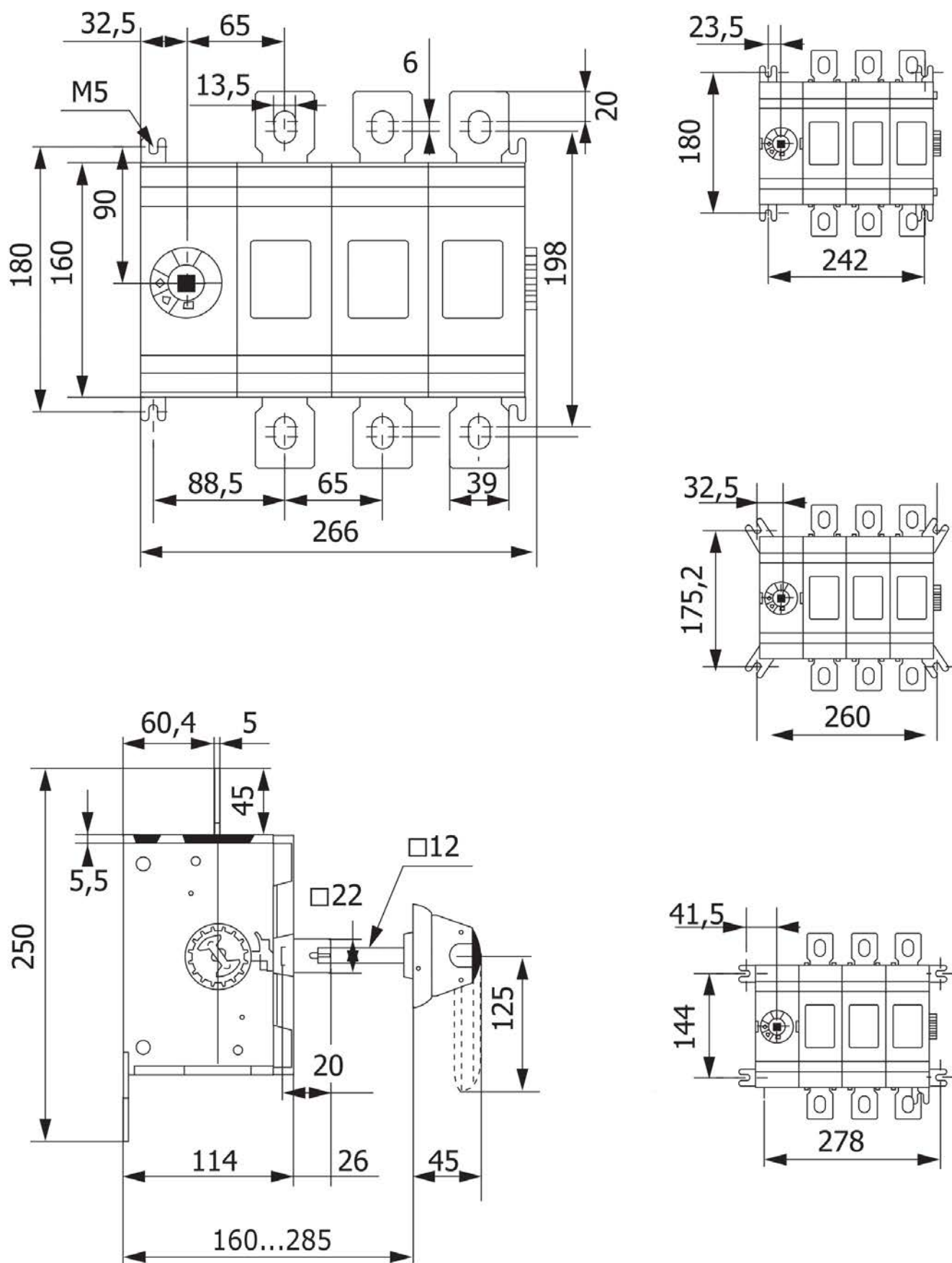
Рис. 7 – Габаритные и установочные размеры рубильников 630-800А 3Р
