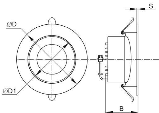
Рисунок 1 – Габаритные размеры ДВО 1811 PRO – ДВО 1813 PRO
