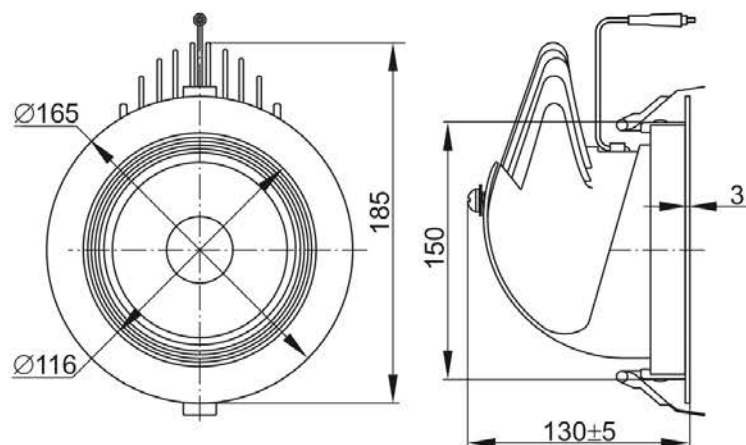
Рисунок 2 – Габаритные размеры ДВО 1822 PRO
