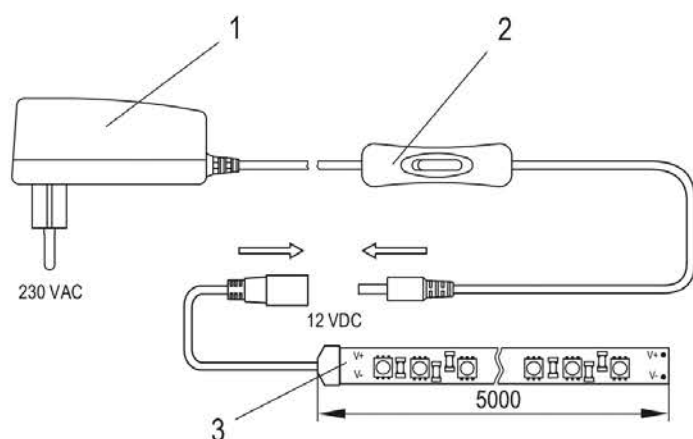
Рисунок 13 – Подключение LSR1-1-060-20-1-2XD12-S3
