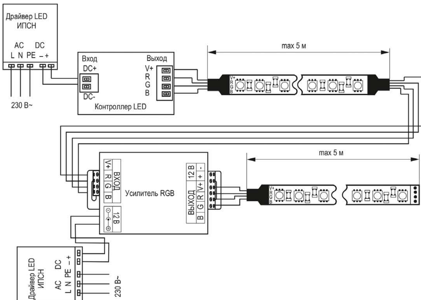
Рисунок 10 – Схема последовательного подключения RGB-усилителя
